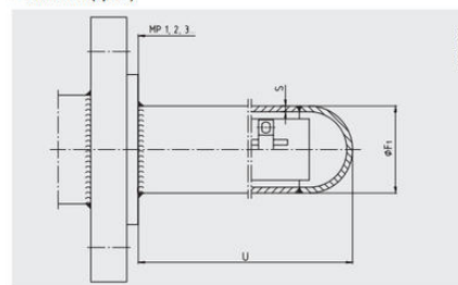
■ Thermowell (option)
