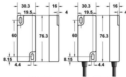
ACTUATOR
