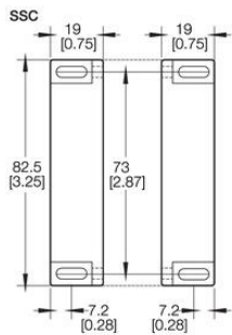
ACTUATOR
