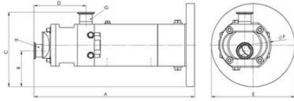
Mät HYDRSPIN Extended kompaktkonrad (mm)
