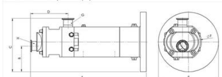
Měří HYGHSPIN Extended kompaktníverad (mm)
