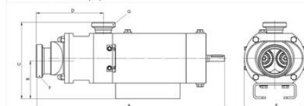
Měří HYGHSPIN Extended 81 axel (mm)
