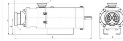
Mått HYGHSPIN full axel (mm)
