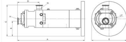
Mått HYGHSPIN kompaktmodell (mm)
