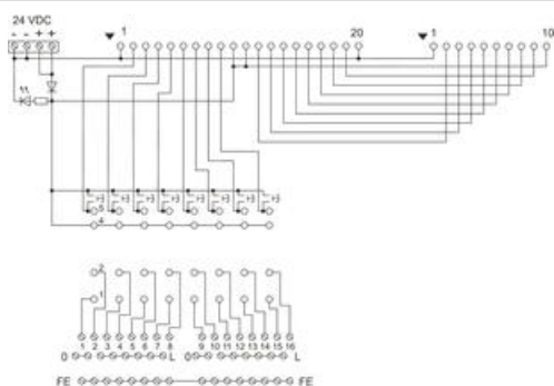
Základní deska pro vstupní relé
