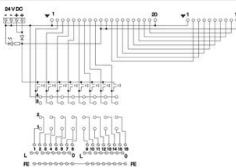
Základní deska pro výstupní relé
