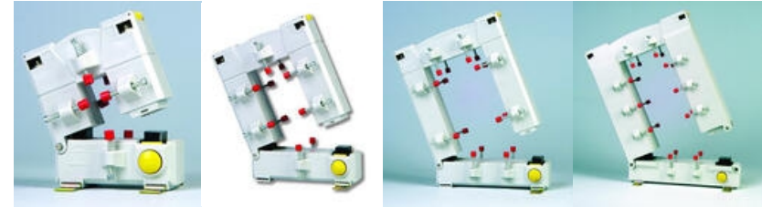
Klešťové proudové transformátory
