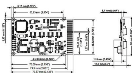
Figure 7.1. ISCM4805 / ISCM8005 dimensions
