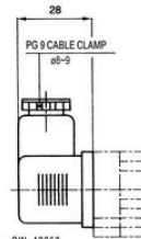
DIN 43650 IP65-ISO4400
