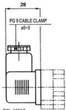
DIN 43650 IP65-ISO4400
