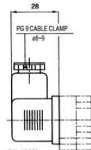
DIN 43850 IP65-ISO4400
