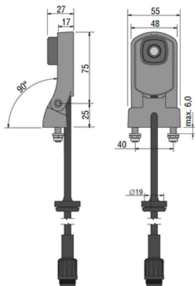
Mått kamera inkl montagefäste (mm)
