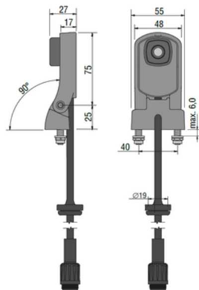
Mått kamera inkl montagefäste (mm)
