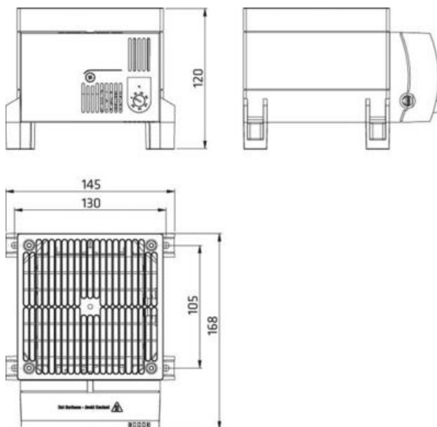
Rozměrové výkresy CS030
