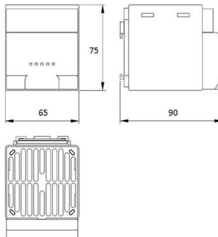
Thermostat KTO011 Heater CS(L) 028
