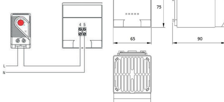
Thermostat KTO011 Heater CS(L) 028
